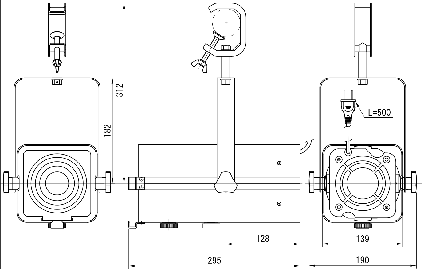
適合パイプφ30~φ48
