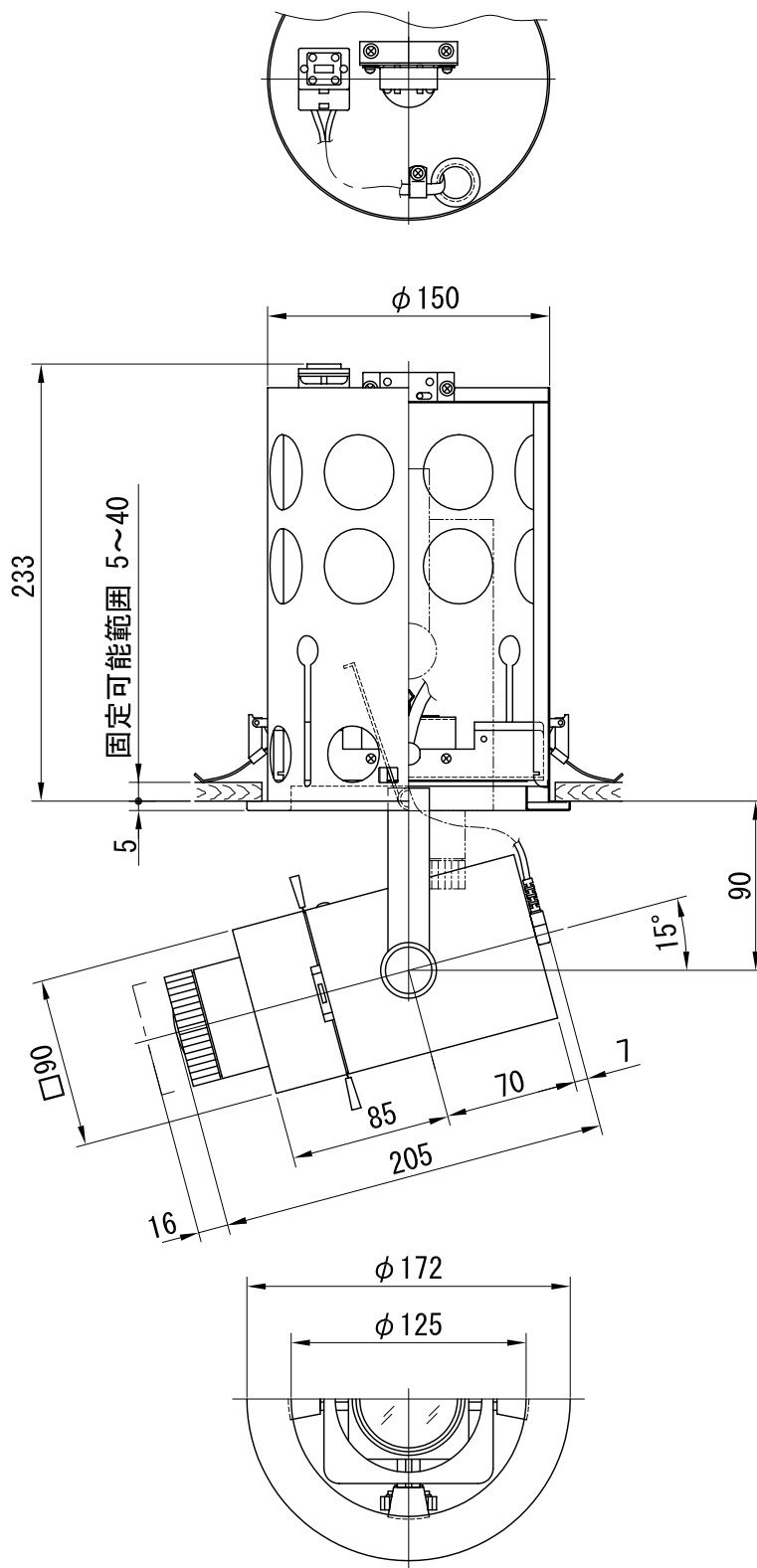
<取付穴寸法>
